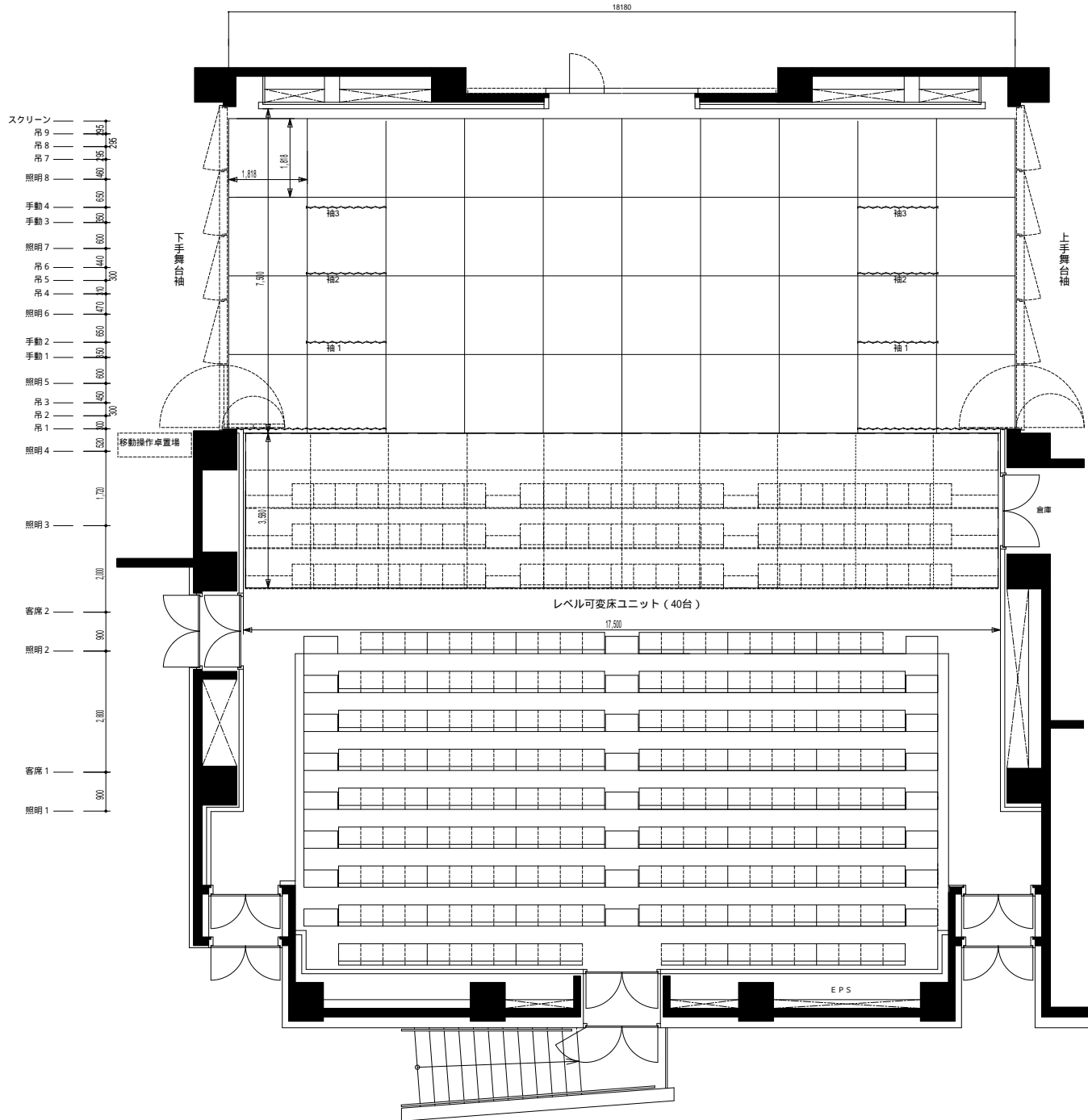
知立市文化会館 (パティオ池鯉鮒) 花しょうぶホール (小ホール) 平面図 (S : 1/100)
