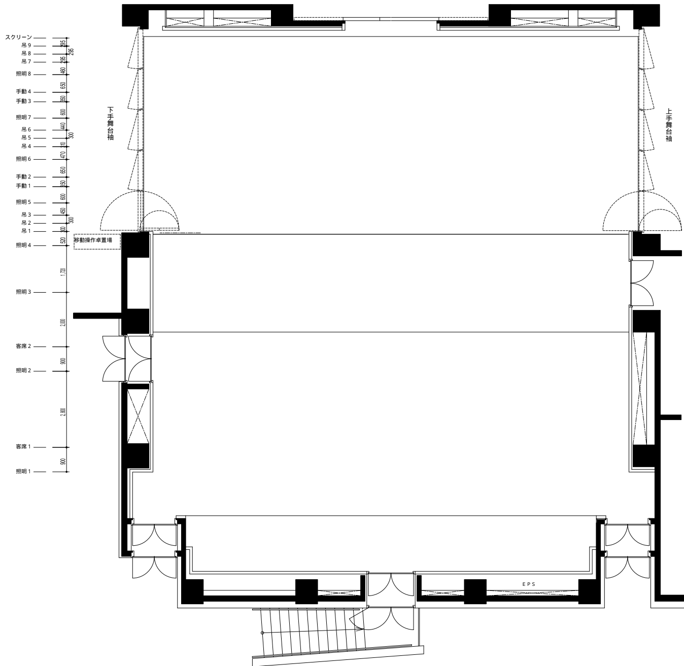
知立市文化会館 (パティオ池鯉鮒) 花しょうぶホール (小ホール) 平土間平面図 (S : 1/100)
